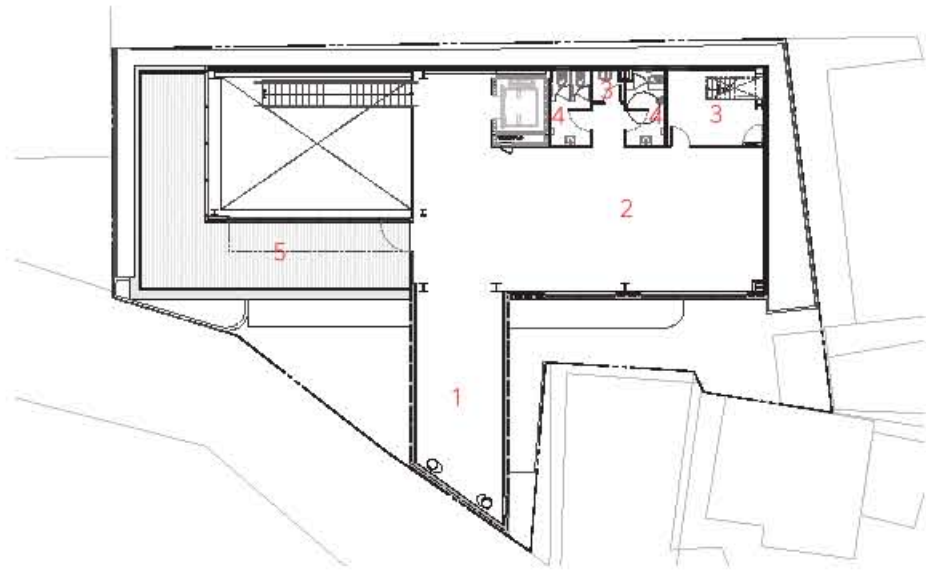
2층 평면도
