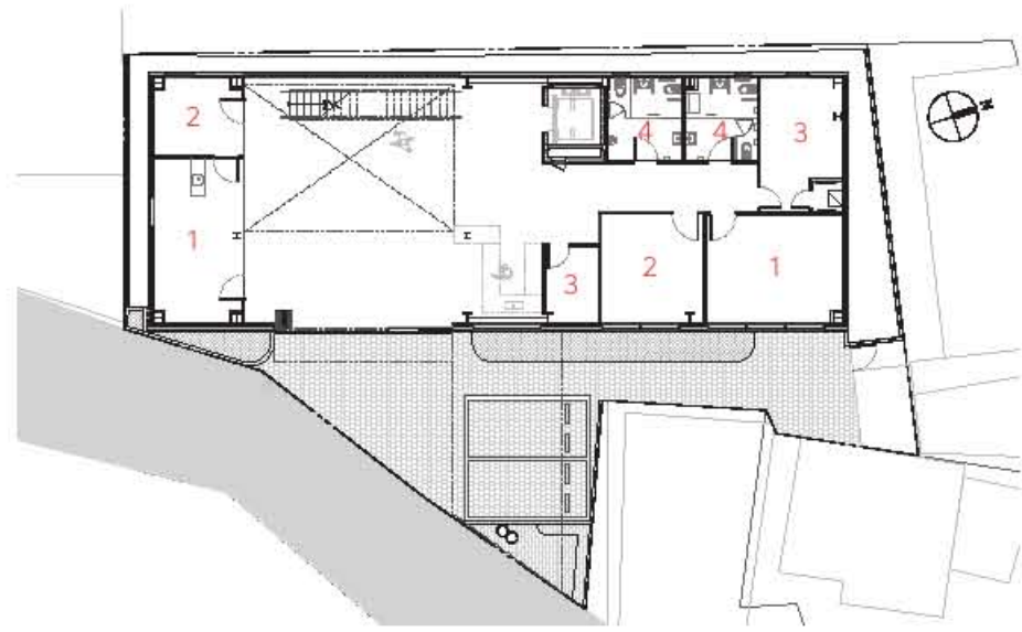
1층 평면도
