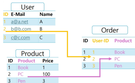
(그림 1) MySQL 구조 예시
