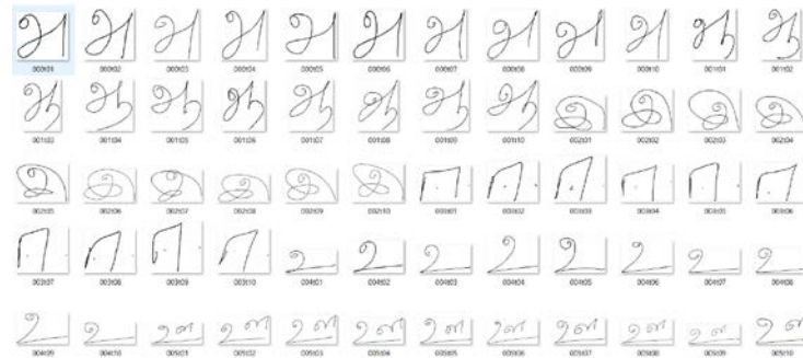
Fig. 4. Tamil Dataset
