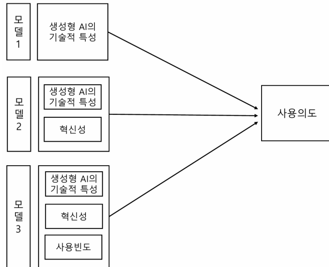
〈그림 1〉 연구모형
