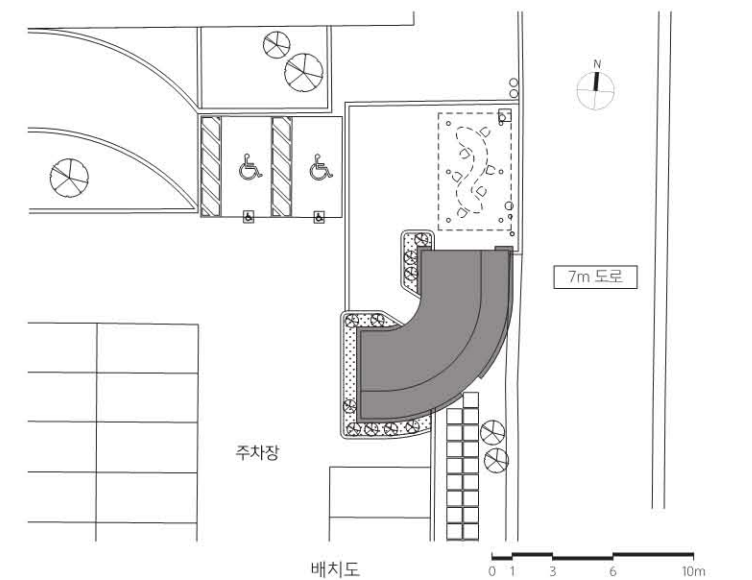
배치도 0 1 3 6 10m
