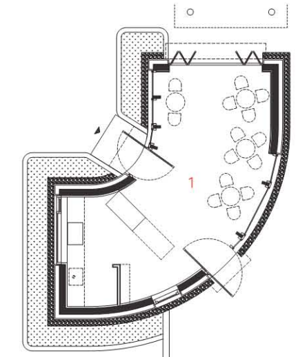
1층 평면도 0 1 3 6m
