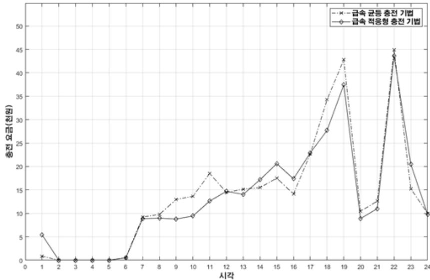
(그림 10) 제안한 급속 적응형 충전 전력 분배 기법의 시간별 충전 요금 모의실험 결과 (Figure 10) Results of simulation of charging fee by time zone using the proposed fast-adaptive charging power distribution technology
