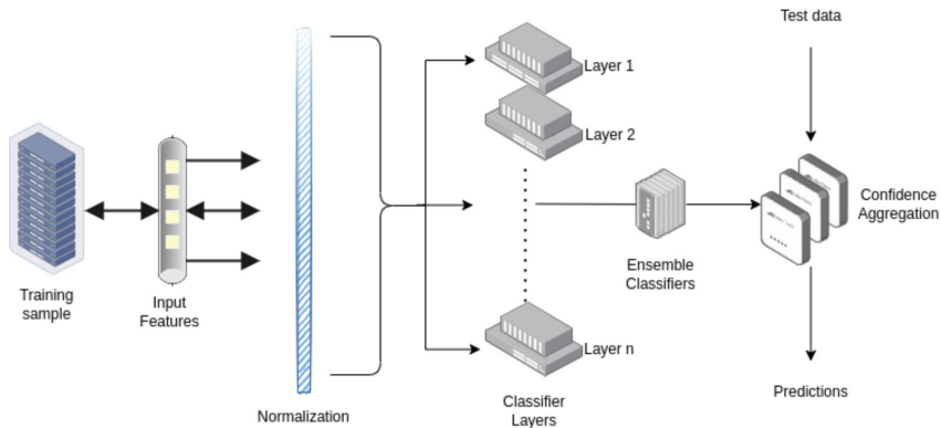
(그림 2) 제안 네트워크
