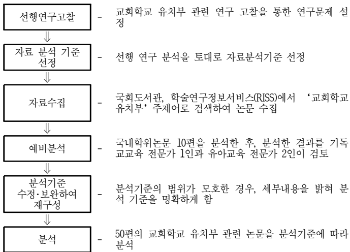
[그림 1] 연구절차
