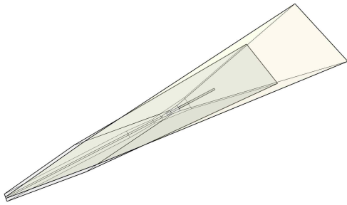
Fig. 5. OAS 비교(짙은 색: SBAS APV-I, 연한 색: ILS CAT-I)
