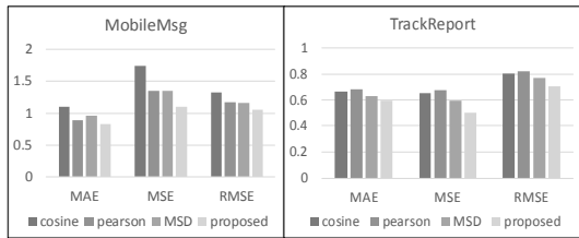
(그림 3) 사용자 기반 CF에서 다른 디스턴스를 활용한 방법과 성능 비교 (Figure 3) Performance comparison with different distance metrics in user-based CF
