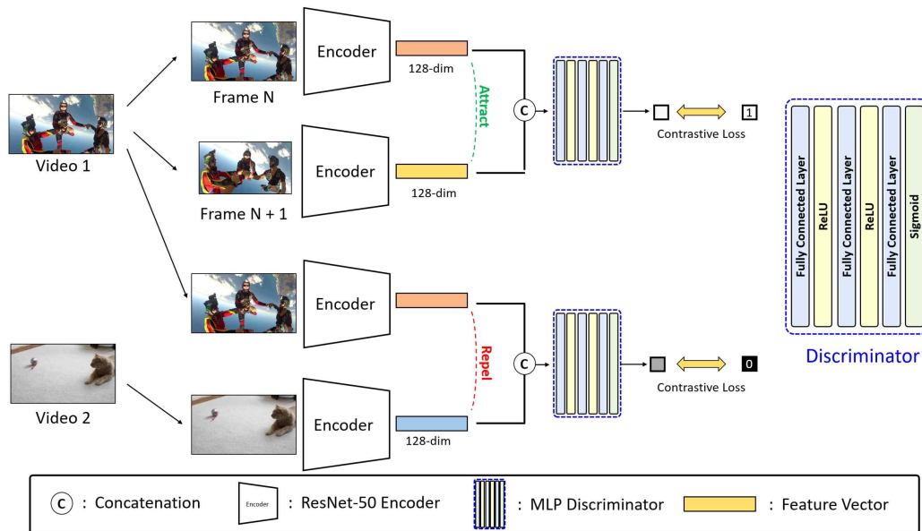
그림 1. 제안하는 대조적 학습 모듈(왼쪽)과 판별기 상세 구조(오른쪽) Fig. 1. Entire structure of the proposed contrastive learning module(left) and details of the discriminator(right)
