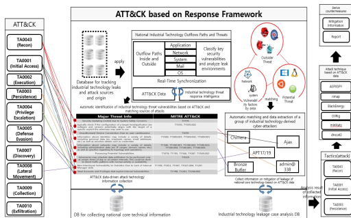
[그림 1] ATT&CK Data 기반의 산업기술 유출방지용 프레임워크 체계화 설계
