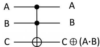
Fig. 2. Toffoli Gate
