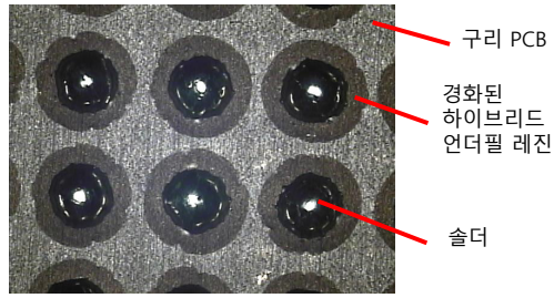
그림 11 하이브리드 언더필 리플로우 공정 후 표면 사진
