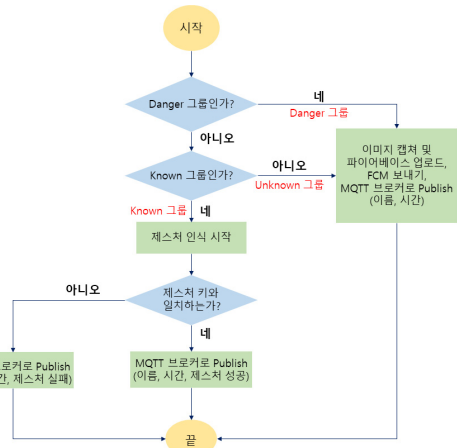
그림 4. 얼굴과 제스처 인식 알고리즘 Fig. 4. Algorithm for recognition of face and hand gesture
