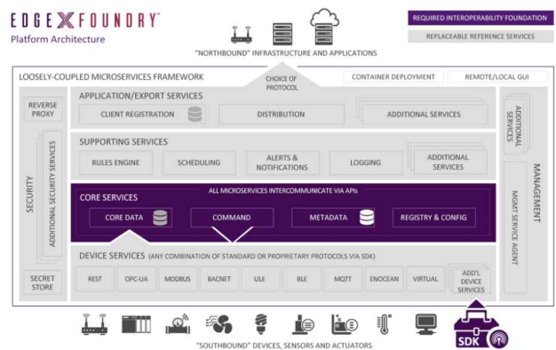
그림 4. EdgeX의 아키텍처
