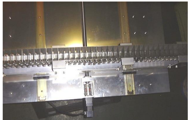
Fig. 11. 40 array horns
