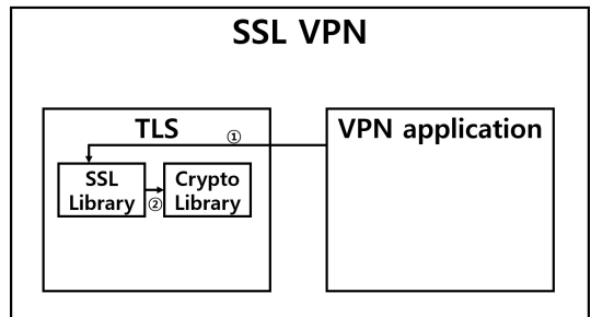
(그림 3) SSL VPN의 암호알고리즘 호출 구조
