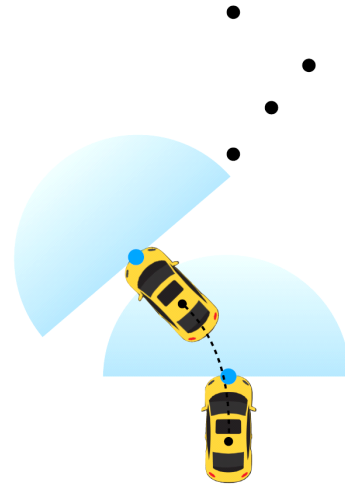
그림 1. 차량용 전방 관측 영상레이다의 운용상황 Fig. 1. Forward-looking imaging radar operation geometry with a vehicle.
