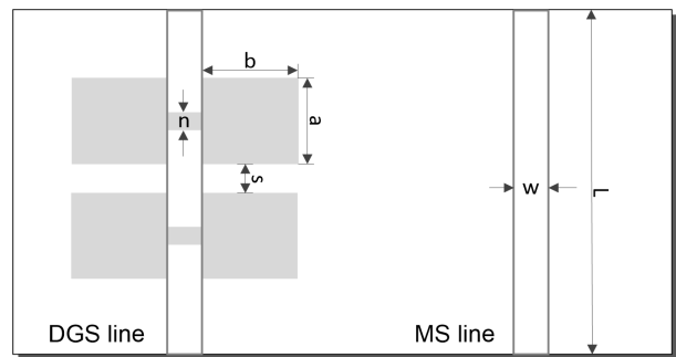
그림 3. 결함접지구조 위상지연 전송선로와 기존 마이크로 스트립 전송선로 비교 Fig. 3. Comparison of a DGS phase delay transmission line and a conventional microstrip transmission line.
