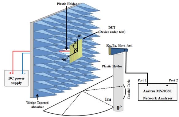
그림 5. 수직입사일 때 흡수율을 측정하기 위한 실험 환경 도시도
