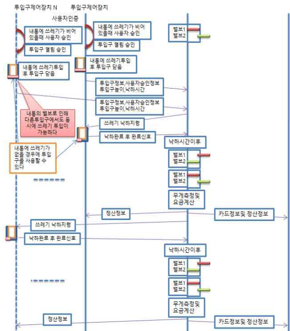
Fig. 4. non-Interlock
