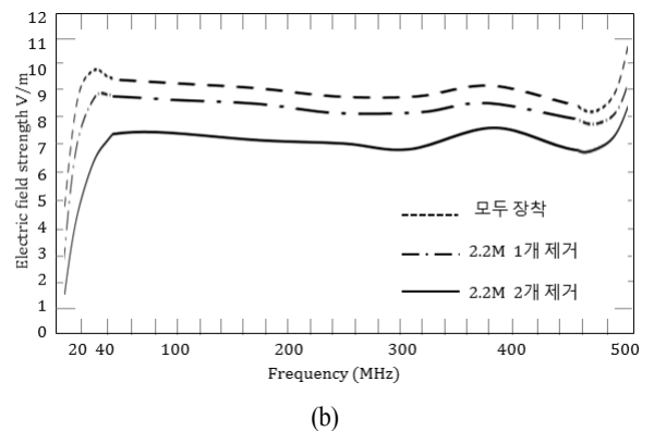
그림 2. 다이폴에 저항로드를 통한 감도 개선 Fig. 2. Sensitivity enhancement with resistor load at dipole.
