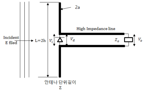
그림 1. 전기장 프로브의 개념도 Fig. 1. Block diagram of electric-field probe.
