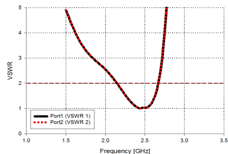
(b) VSWR
