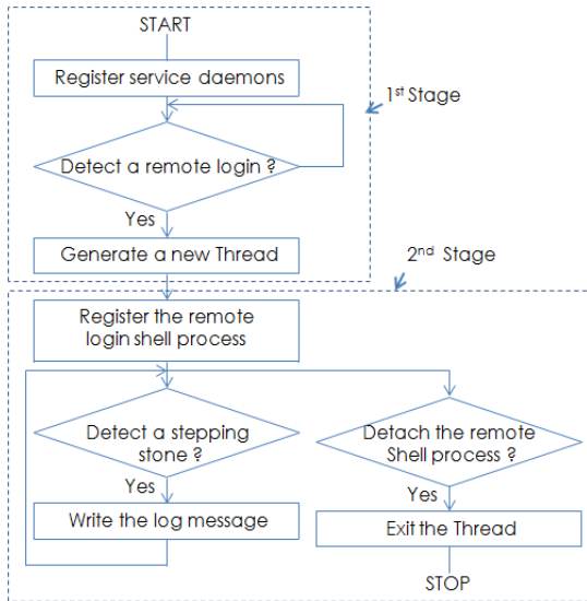
그림 4. 기본 알고리즘 Fig. 4. Basic algorithm
