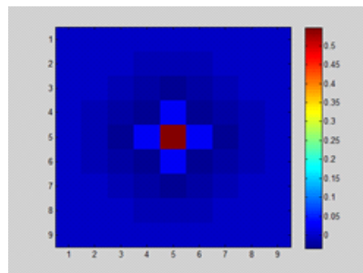
그림 5. 9×9 크기 DOG 마스크 Fig. 5. 9×9 Size DOG Mask
