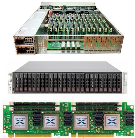
(그림 10) Boston Viridis 서버와 Calxeda EnergyCard
