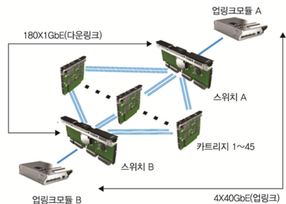
(그림 13) HP Moonshot 1500 시스템 네트워크
