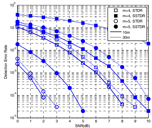
그림 4. 고장위치에 따른 탐지 기법별 오탐지율 Fig. 4. Detection error rates with different fault locations and detection methods
