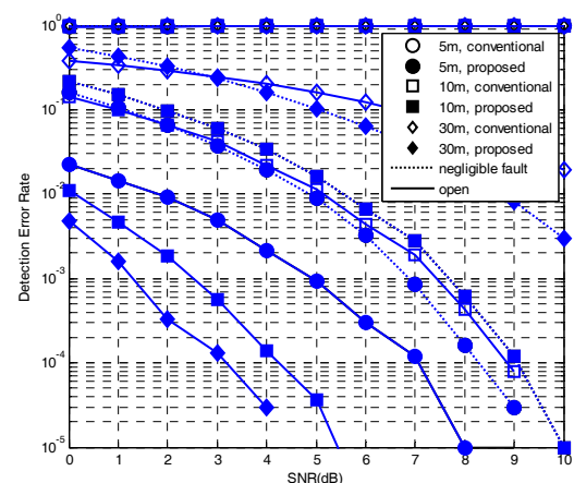
그림 9. 고장탐지 제거 기법별, 고장유형별 오탐지율 Fig. 9. Detection error rates of the conventional and proposed SSTDR
