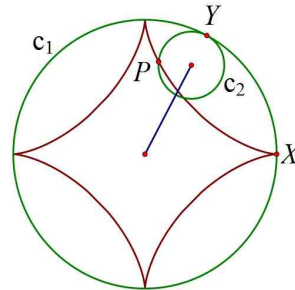
[그림 25] 하이포사이클로이드의 접선 탐색 과정 2 [Fig. 25] Process exploring tangent line of hypocycloid 2
