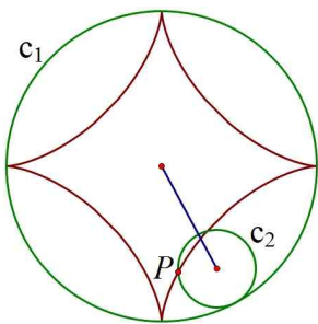
[그림 20] 하이포사이클로이드 [Fig. 20] Hypocycloid
