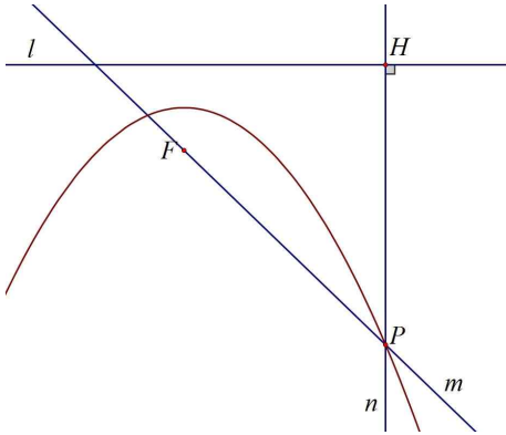
[그림 1] 포물선의 접선 탐색 과정 1 [Fig. 1] Process exploring tangent line of parabola 1
