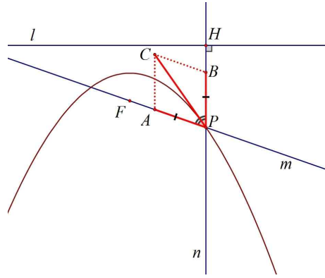
[그림 3] 포물선의 접선 탐색 과정 3 [Fig. 3] Process exploring tangent line of parabola 3
