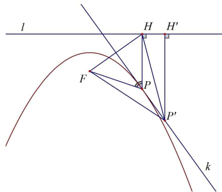
[그림 4] 포물선의 접선 탐색 과정 4 [Fig. 4] Process exploring tangent line of parabola 4
