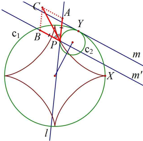
[그림 26] 하이포사이클로이드의 접선 탐색 과정 3 [Fig. 26] Process exploring tangent line of hypocycloid 3
