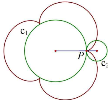
[그림 27] 에피사이클로이드의 접선 탐색 과정 1 [Fig. 27] Process exploring tangent line of epicycloid 1
