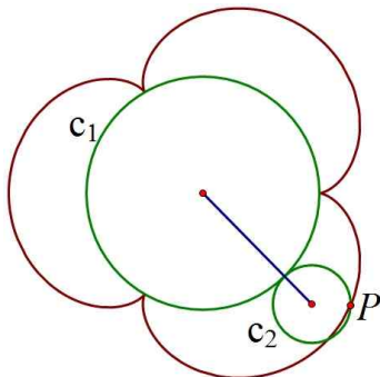
[그림 21] 에피사이클로이드 [Fig. 21] Epicycloid
