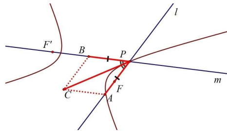
[그림 14] 쌍곡선의 접선 탐색 과정 3 [Fig. 14] Process exploring tangent line of hyperbola 3
