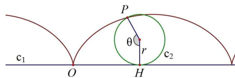
[그림 22] 사이클로이드의 접선 탐색 과정 2 [Fig. 22] Process exploring tangent line of cycloid 2
