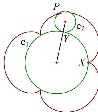
[그림 28] 에피사이클로이드의 접선 탐색 과정 2 [Fig. 28] Process exploring tangent line of epicycloid 2
