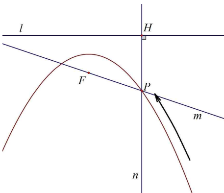
[그림 2] 포물선의 접선 탐색 과정 2 [Fig. 2] Process exploring tangent line of parabola 2
