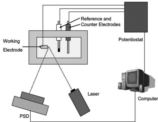
그림 5 캔틸레버를 이용한 수질내 크롬, 납 등의 중금속 이온의 검출(오크리지 국립연구소)
