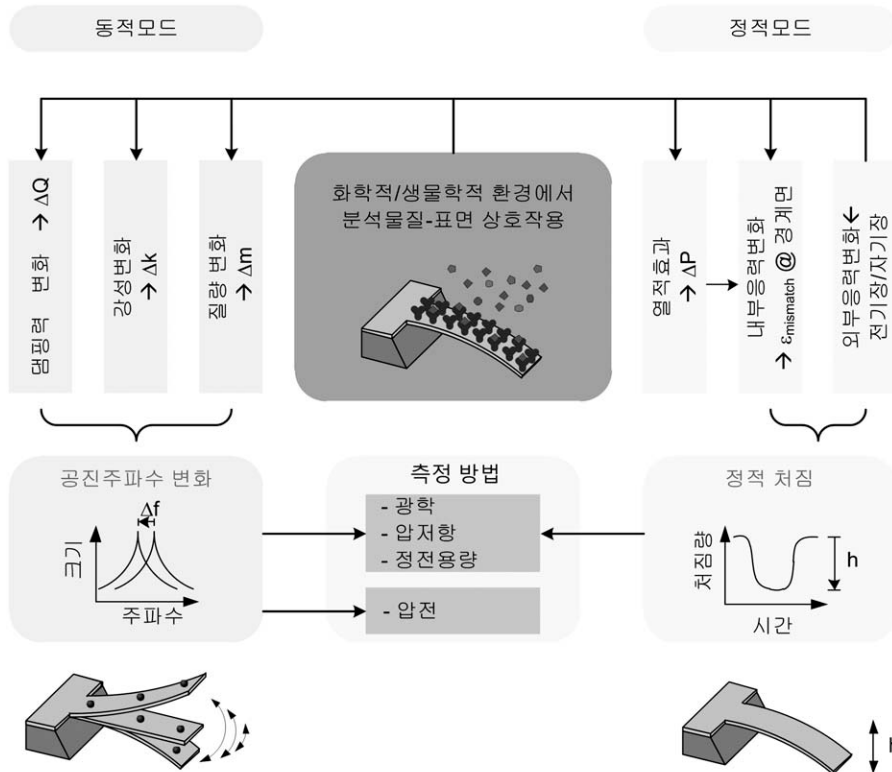
그림 2 캔틸레버 센서의 작동 원리
