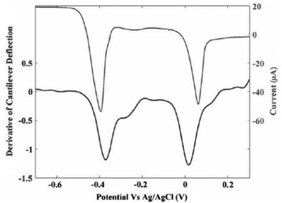
그림 5 캔틸레버를 이용한 수질내 크롬, 납 등의 중금속 이온의 검출(오크리지 국립연구소)
