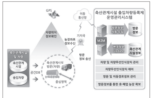
〈축산시설 출입정보수집시스템 구성도〉
