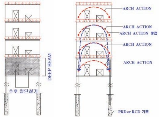
그림 6. 최하층벽체 전담방식 그림 7. 적층 아치 거동방식
