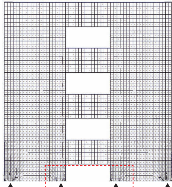
그림 10. 전체 응력흐름도(Arch Action)
