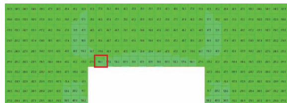
그림 12. 최대 응력(Stress) \sigma_{xx \max} = 186.1 \text{ kN/m}^2
