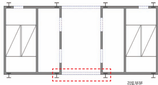
그림 9. 코어 평면+H형강 기둥배치
