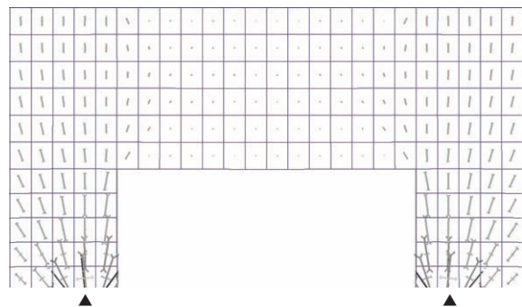
그림 11. 부분 응력흐름도(Arch Action)
