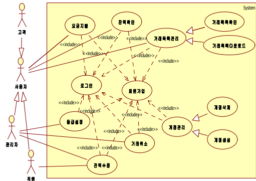
그림 2. '온라인 뱅킹 시스템'을 위한 유스케이스 모델 Fig 2. Use case model for on-line banking system
