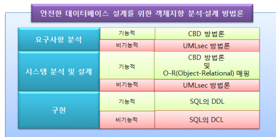
그림 1. 제안한 '안전한 데이터베이스 설계를 위한 객체지향 분석·설계 방법론'의 과정
