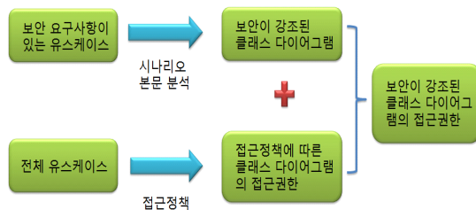
그림 3. 접근정책에 따른 보안이 강조된 클래스 다이어그램의 생성과정 Fig 3. Creating process of security emphasized class diagram depending on access policy
