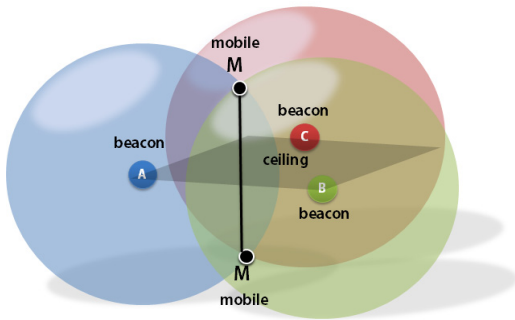
그림 5. 구의 방정식 기반 3차원 위치좌표 계산 개념 Fig. 5. Concept of calculation of 3D location coordinates based on 3 sphere equations.
