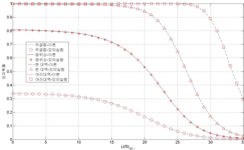
그림 3. C/N_0 가 40 dB-Hz, 오경보확률이 10^{-3} , 위성과 수신기의 가시선이 확보되는 환경에서 하나의 확산신호만 있는 ‘무결합’과 M_1 = M_{I,1} = 2 인 ‘동위상’ 결합, M_1 = 4, M_{I,1} = 2 인 ‘한 대역’ 결합, CH = 2, M_1 = M_2 = 4, M_{I,1} = M_{I,2} = 2 인 ‘여러대역’ 결합일 때, 입력 광대역 전파방해신호 대 신호 전력비에 따른 검파확률 Fig. 3. Detection probabilities according to input jamming to signal power ratio from 0 to 35 dB when the false alarm probability is 10^{-3} ( C/N_0 = 40 dB-Hz)
