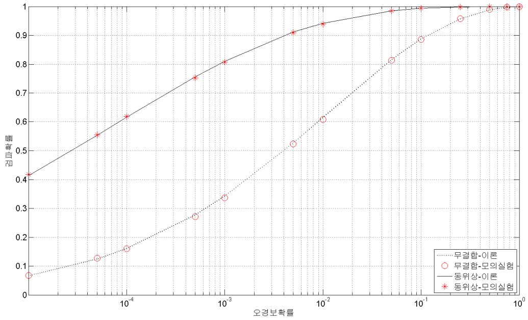
그림 2. 광대역 전파방해가 없고 C/N_0 가 40 dB-Hz인 위성과 수신기의 가시선이 확보되는 환경에서 하나의 확산신호만 있는 ‘무결합’과 M_1 = M_{I,1} = 2 인 ‘동위상’ 결합일 때, 오경보확률에 따른 검파확률 Fig. 2. Detection probabilities according to false alarm probability when broadband jamming is free in normal receiving environment ( C/N_0 = 40 dB-Hz)
