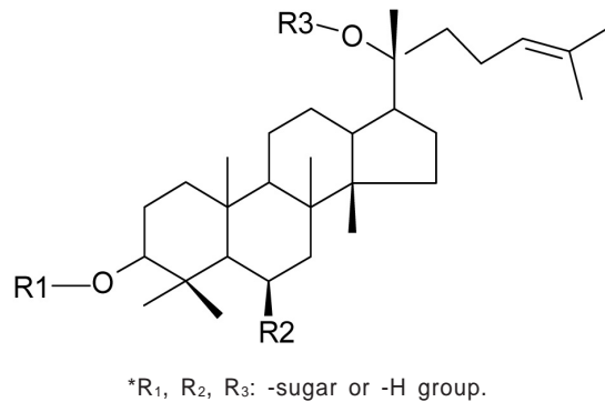
Fig.1. 고려인삼 사포닌의 구조
