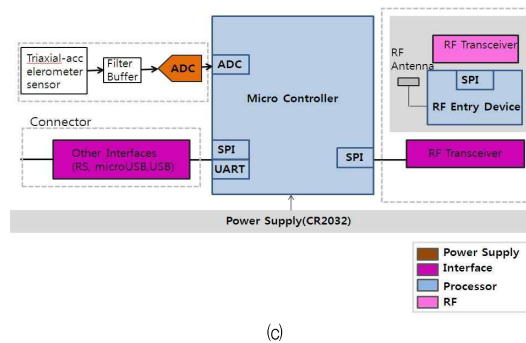
(a) 인체 활동 모니터링을 위한 전체 구성도 (b) 제안된 인체 활동 측정 모듈시스템 (c)시스템의 블록도 그림 1. 인체 활동 모니터링 시스템의 구성도 및 블록도 (a) configuration for monitoring human activities (b) Measurement module system proposed human activities (c) Block diagram of the system Fig. 1. a block diagram of the configuration of monitoring system
