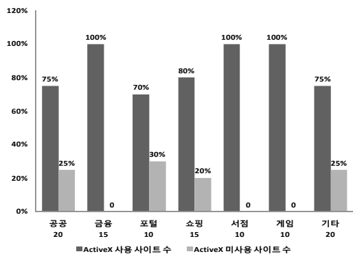
그림1 민간 100대 사이트 ActiveX의 사용현황 Fig. 1. 100 Sites Private Agencies use of ActiveX
