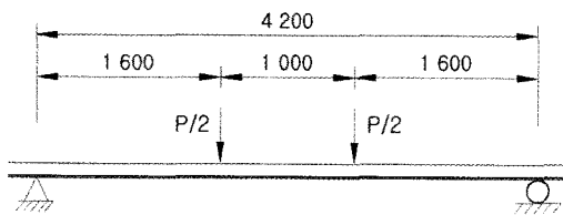
그림 1. 경계조건 및 하중조건
