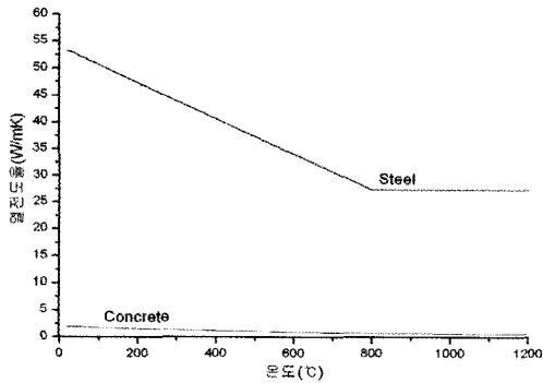
그림 7. 강재 및 콘크리트의 열전도율(Eurocode 4 Part1.2)
