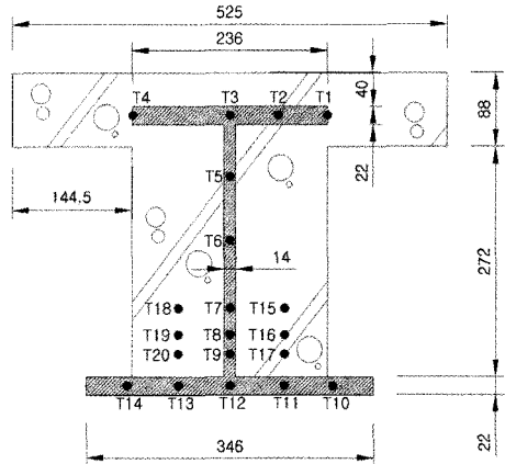
그림 2. 시험체 단면형상 및 온도측정위치
