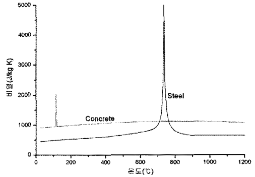
그림 8. 강재 및 콘크리트의 비열(Eurocode 4 Part1.2)
