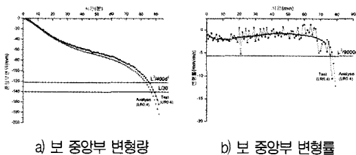
그림 13. 구조해석 결과 비교
