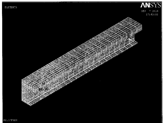
그림 6. 1/4모델 형상
