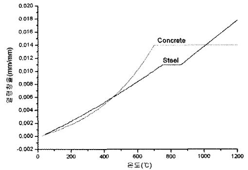
그림 9. 강재 및 콘크리트의 열팽창율(Eurocode 4 Part1.2)
