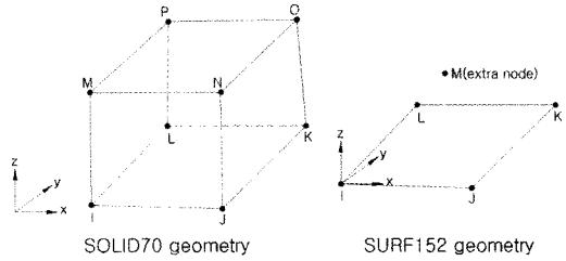
그림 5. 요소형상
