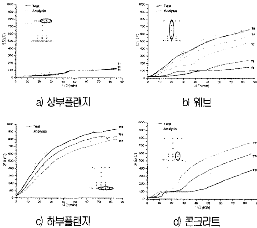
그림 12. 열전달해석 결과 비교
