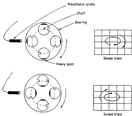
그림 2.19 Orbital Plot에서 Keyphasor 신호에 의한 위상각 정보
