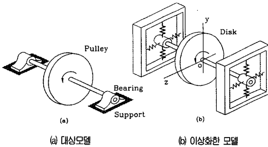
그림 2.3 이방성을 갖는 베어링에 의해 지지되는 회전체
