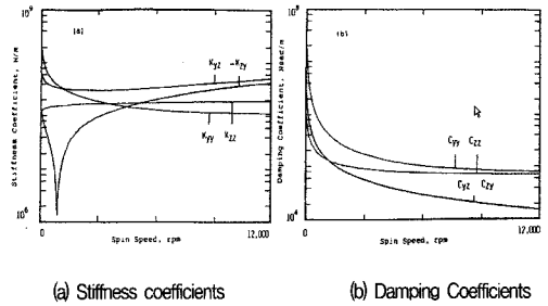
그림 2.5 저널 베어링의 회전속도에 대한 동적계수 변화
