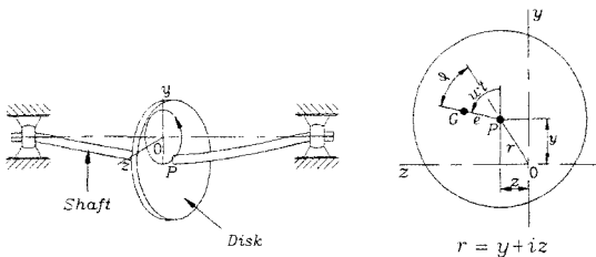
그림 2.1 단순회전체 모형
