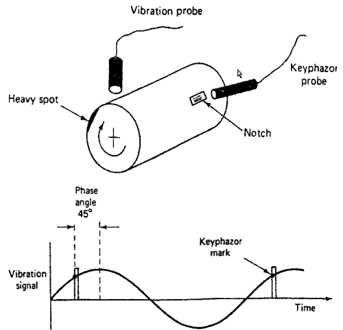
그림 2.14 Keyphasor Probe의 역할
