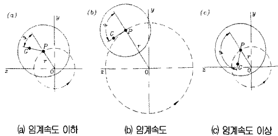
그림 2.2 단순회전체 회전속도에 따른 선회계적
