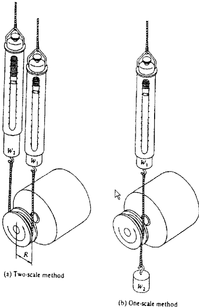
그림 2.15 기계적 토크 측정방법
