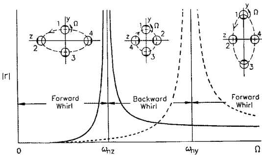
그림 2.4 이방성을 갖는 회전체의 회전속도에 따른 불균형 응답 변화
