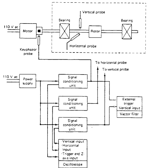
그림 2.18 Orbital Plot에서 Keyphasor 신호를 이용하는 방법
