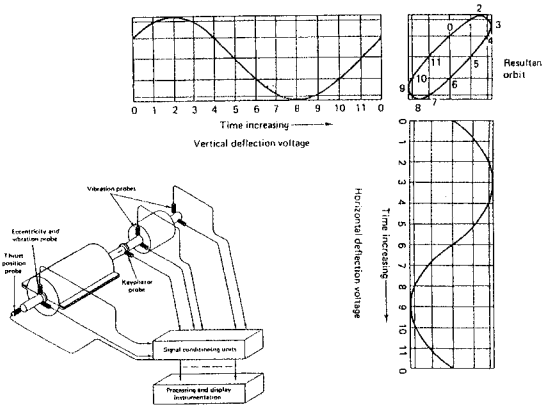
그림 2.17 실측에 의해 Orbital Plot을 구하는 원리
