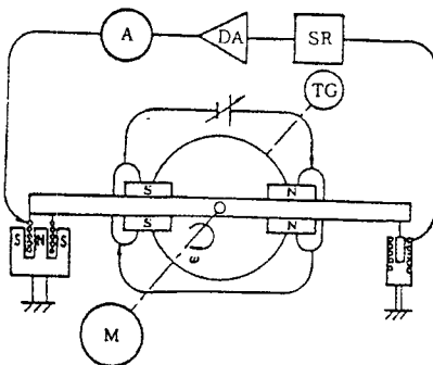
그림 2.16 전자기적 천평원리를 이용한 토크 측정장치
