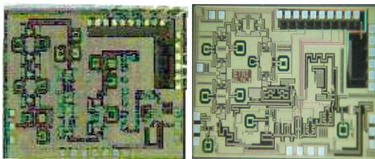
(그림 13) SiGe Ku-대역 상/하향 다기능 MMIC
