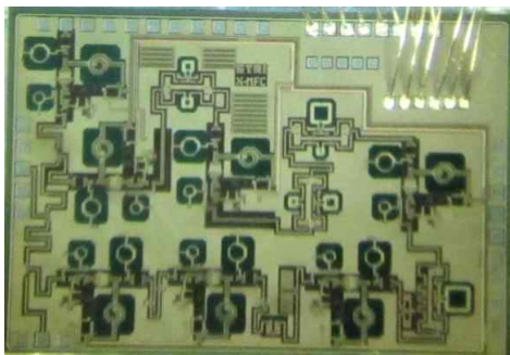
(그림 12) SiGe X-대역 다기능 MMIC
