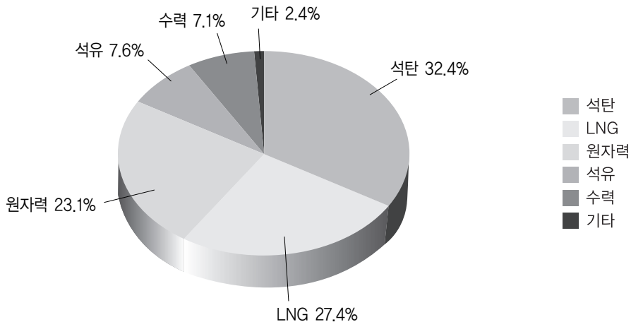
[연료원별 발전설비용량]
