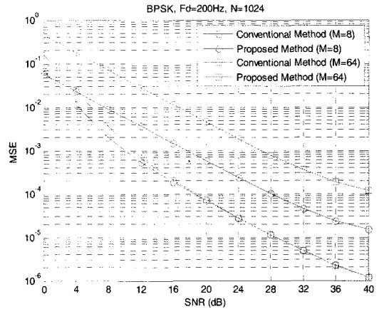
그림 4. 기존 기법과 제안된 기법의 MSE 성능비교 Fig. 4. Comparison of the MSE for different estimation technique
