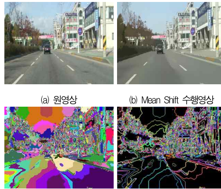
(a) 원영상 (b) Mean Shift 수행영상 (c) 라벨링 영상 (d) 라벨 윤곽영상 그림 2 초기 분할된 결과 영상 Fig. 2 Initial segmentation results
