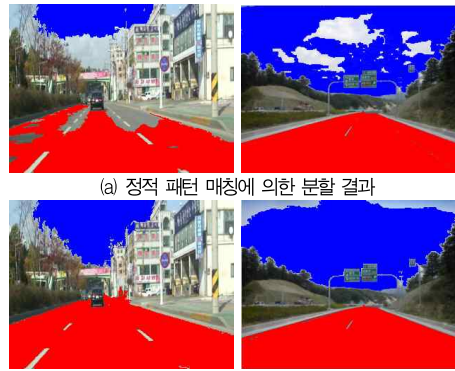
(a) 정적 패턴 매칭에 의한 분할 결과 (b) 적응적 패턴 매칭에 의한 분할 결과 그림 8. 정적인 패턴과 제안된 적응적인 패턴 매칭에 의한 영상분할 결과 영상 Fig. 8. Segmentation results by using a static-pattern matching and the proposed adaptive-pattern matching method
