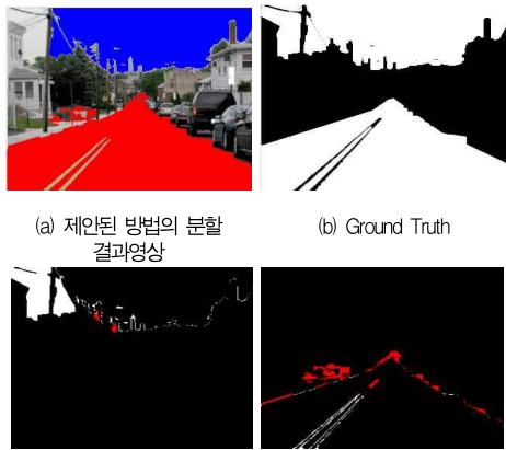
그림 7. 제안된 방법의 오류분석 Fig. 7. Error analysis of the proposed method
