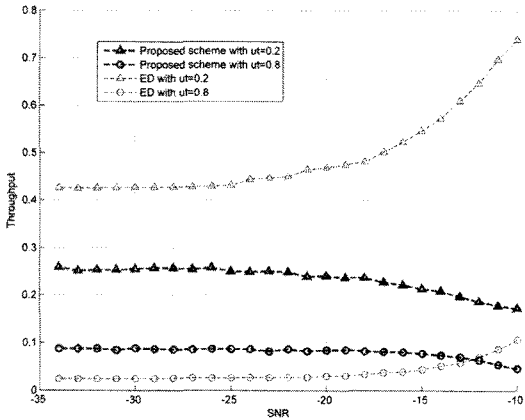
(그림 9) AWGN+레이레이 채널에서 처리율 성능 비교
