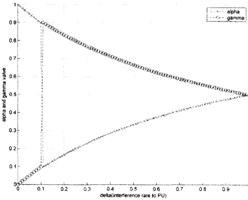
(그림 6) \Delta = 1 일 때, \delta 에 따른 \alpha , \gamma 의 값
