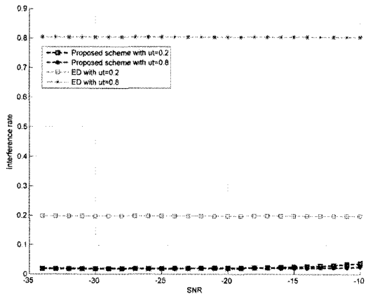
(그림 10) AWGN+레이레이 채널에서 간섭률 성능 비교
