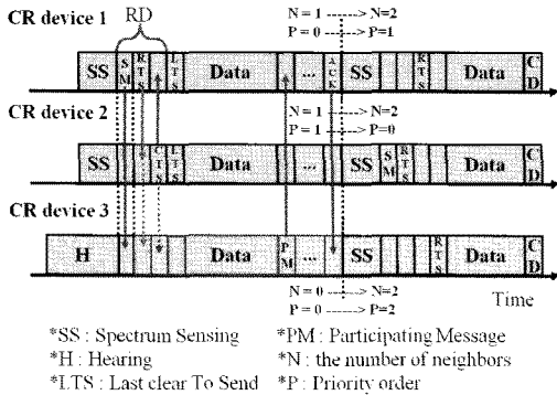
(그림 4) 미니 슈퍼프레임의 데이터 전송과정
