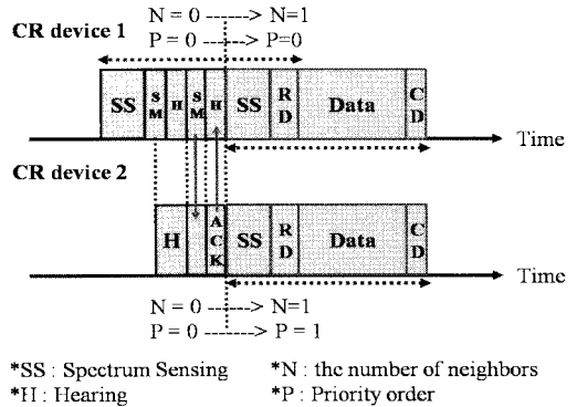
(그림 3) 미니 슈퍼프레임의 동기화 과정(2)
