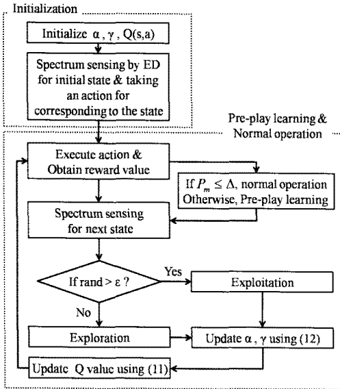
(그림 7) Q-learning 기반 채널접근기법의 전체 흐름도
