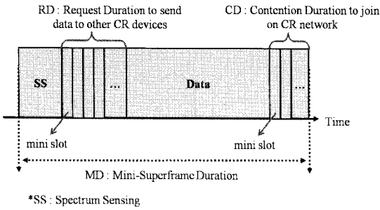
(그림 1) 미니 슈퍼프레임의 구조
