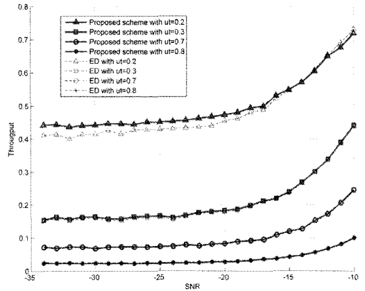
(그림 8) AWGN 채널에서의 처리율 성능 비교
