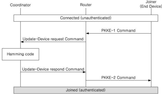
그림 4. 제안하는 SmartGrid ZigBee 네트워크에서의 새로운 디바이스의 합류 과정
