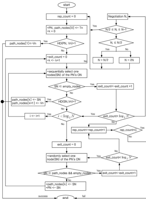
그림 8 제안한 경로 구축 알고리즘 Fig 8. Proposed Certificate path algorithm.
