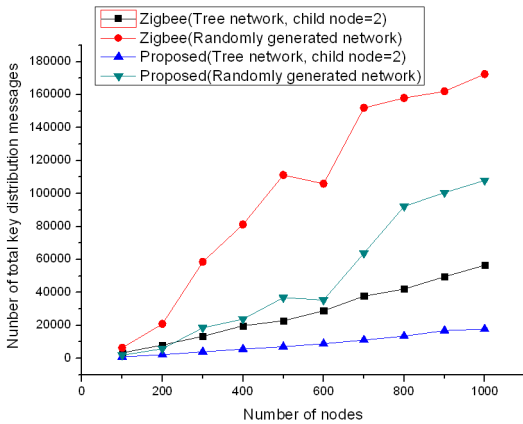
그림 9. 제안하는 ZigBee 네트워크와 기존의 ZigBee 네트워크에서 키 분배를 하기 위한 메시지 개수 비교
