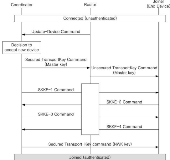
그림 3. 기존 ZigBee 네트워크에서의 새로운 디바이스의 합류 과정 Fig 3. Key establishment process in ZigBee network.
