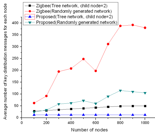
그림 11. 제안하는 방식과 기존 ZigBee 방식에 따라 신뢰 센터를 제외한 노드에서 키 분배를 위해 전송하는 메시지의 평균 개수 비교
