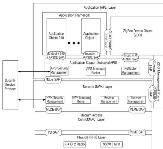
그림2 ZigBee 스택 구조 Fig 2. Architecture of ZigBee stack.
