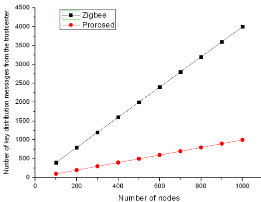
그림 10. 제안하는 방식과 기존 ZigBee 방식에 따라 키 분배를 위해 신뢰센터에서 전송하는 메시지 개수 비교
