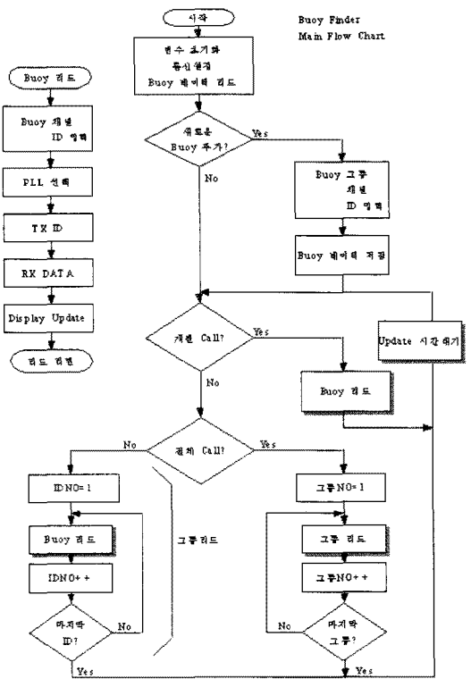
그림 3. 부표탐지기의 S/W 흐름도
