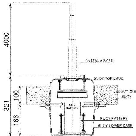
그림 6. 무선부표 기구 설계도
