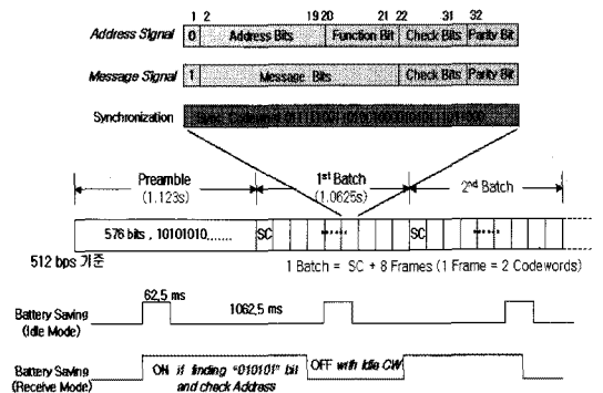
그림 1. 무선부표용 전송신호 포맷
