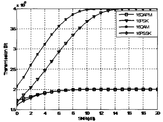
(a) 16-ary AWGN 채널 throughput 성능
