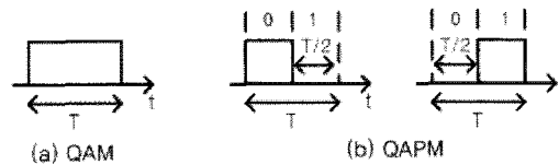
그림 2. QAPM 심볼 구간
