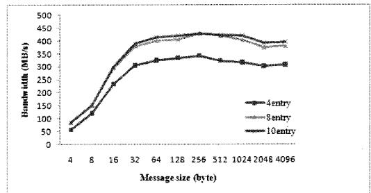
그림 11. 8 대 8 통신 Fig 11. 8 to 8 communication
