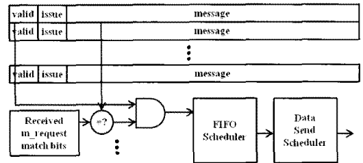
그림 6. 준비 큐 Fig 6. Ready queue
