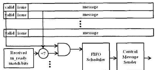
그림 7. 예약 큐 Fig 7. Reserve queue
