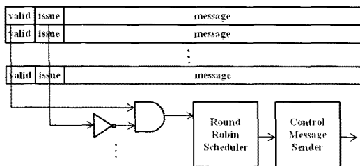
그림 5. 요청 큐 Fig 5. Request queue
