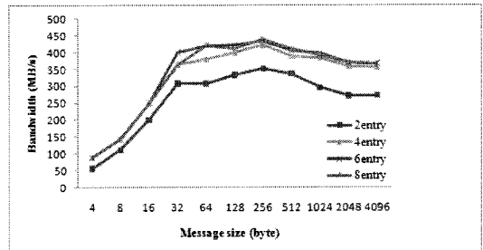
그림 10. 4 대 4 통신 Fig 10. 4 to 4 communication
