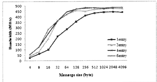
그림 9. 1 대 4 통신 Fig 9. 1 to 4 communication
