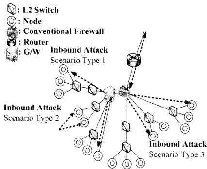
그림 15. 전형적인 방화벽에 대한 네트워크 공격
