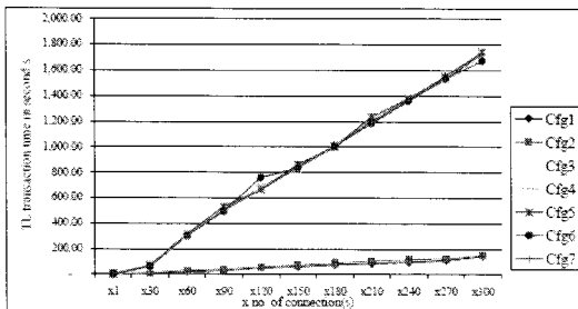
그림 4. HTTP 전체 평균 전송시간 대 연결 수
