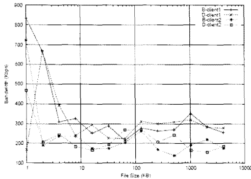
그림 10. 다중 사용자의 NAT 대역폭 사용률
