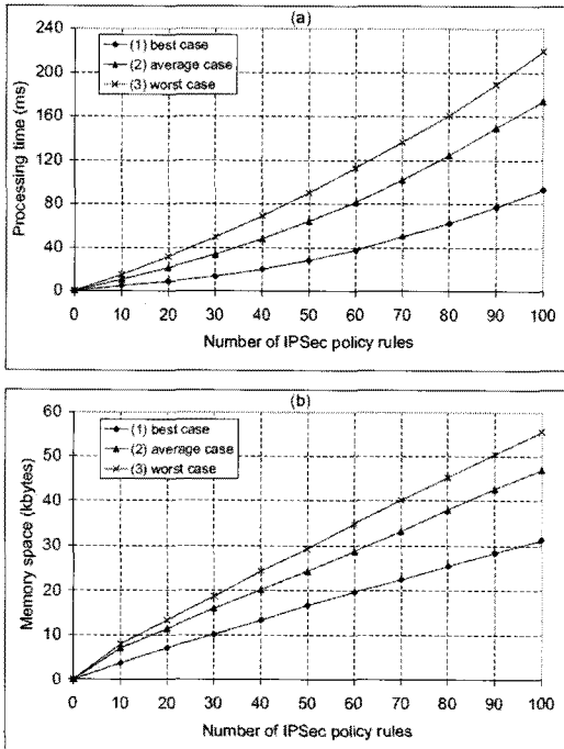
그림 7. IPsec의 내부 정책 수에 따른 수행시간과 메모리 사용량
