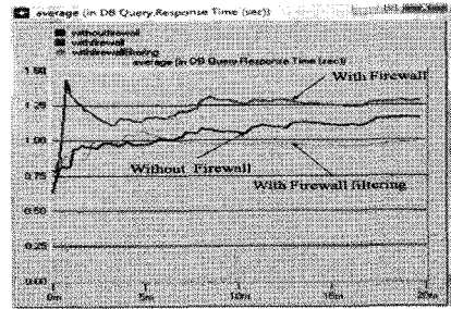
그림 1. HTTP 서버 응답시간
